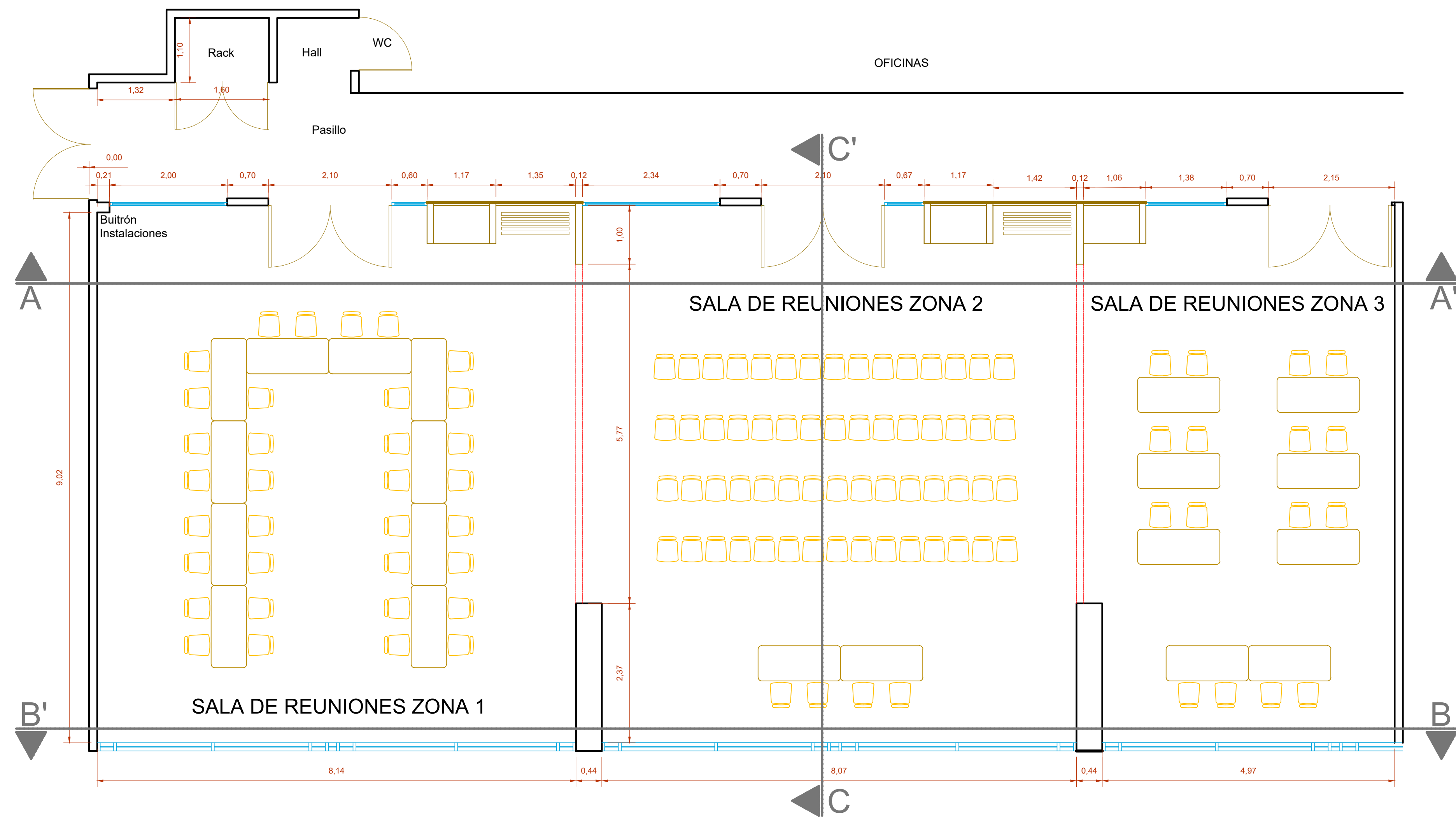
PLANTA GENERAL ESC 1:50
