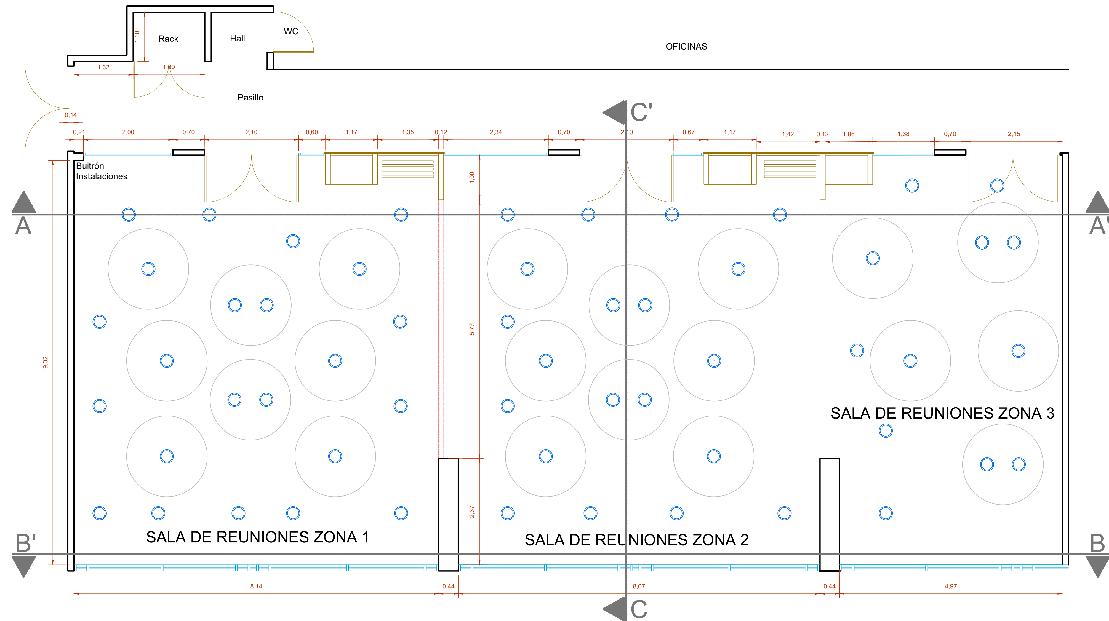
PLANTA DE DISTRIBUCION DE ILUMINACION ESC 1:50
