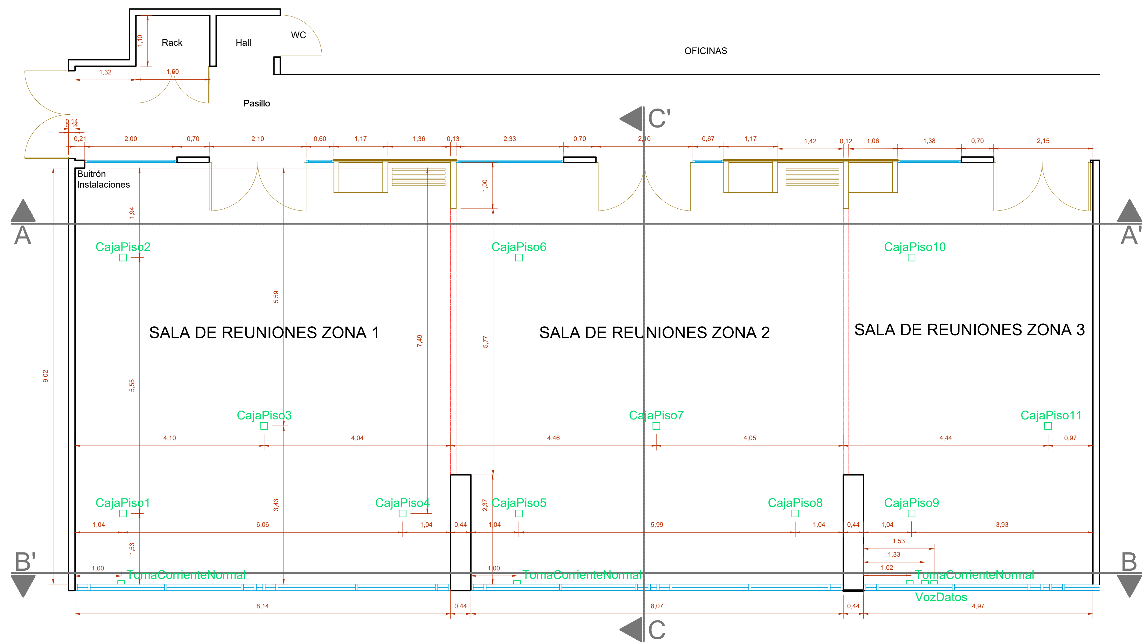
PLANTA DE DISTRIBUCION DE CAJAS DE PISO ESC 1:50
