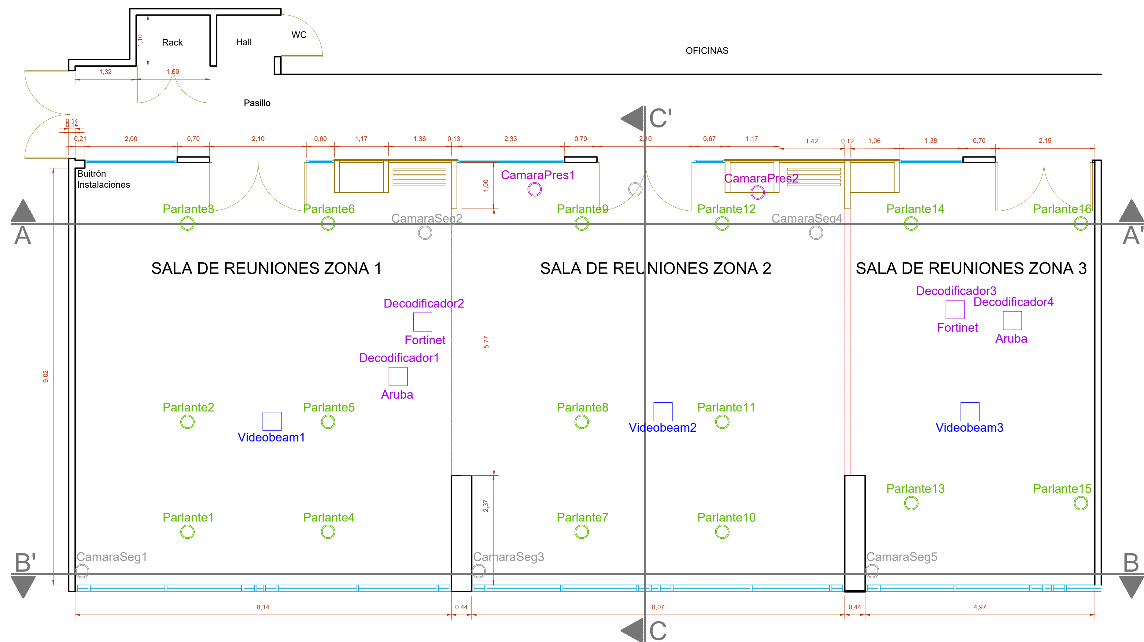
PLANTA DE DISTRIBUCION DE APARATOS DE TECNOLOGIA EN TECHO ESC 1:50
